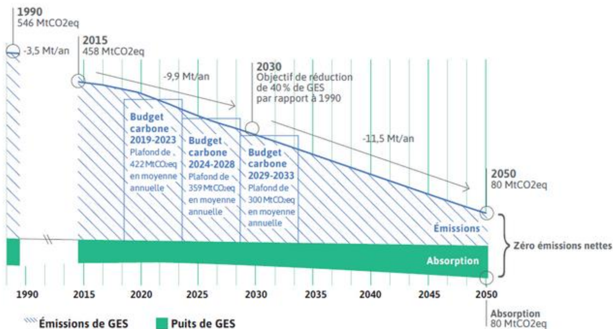
Figure 2. Evolution des émissions et des puits de GES sur le territoire français entre 1990 (en MtCO 2 eq)
